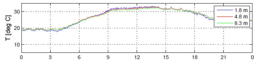
BLLAST Lannemezan site 1 flux GFI 26.06.2011
