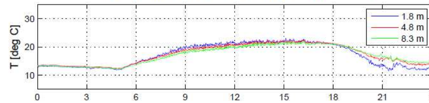
BLLAST Lannemezan site 1 flux GFI 01.07.2011
