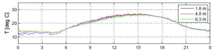
BLLAST Lannemezan site 1 flux GFI 05.07.2011
