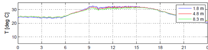
BLLAST Lannemezan site 1 flux GFI 27.06.2011
