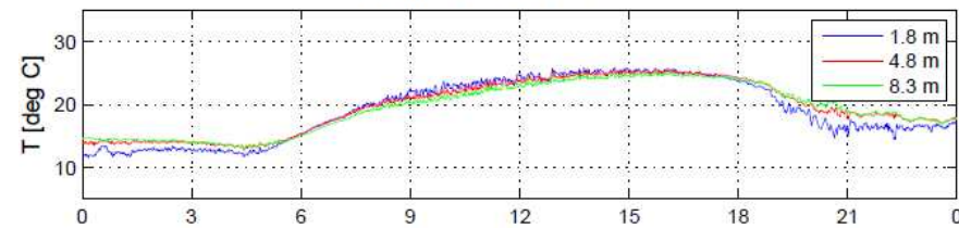
BLLAST Lannemezan site 1 flux GFI 02.07.2011
