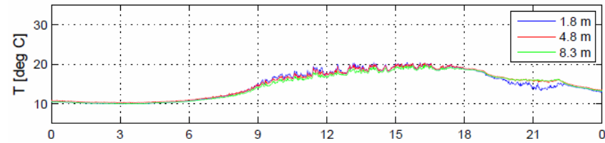
BLLAST Lannemezan site 1 flux GFI 30.06.2011
