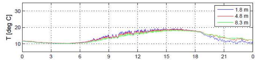
BLLAST Lannemezan site 1 flux GFI 24.06.2011
