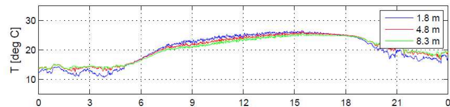
BLLAST Lannemezan site 1 flux GFI 20.06.2011
