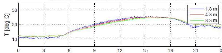
BLLAST Lannemezan site 1 flux GFI 25.06.2011
