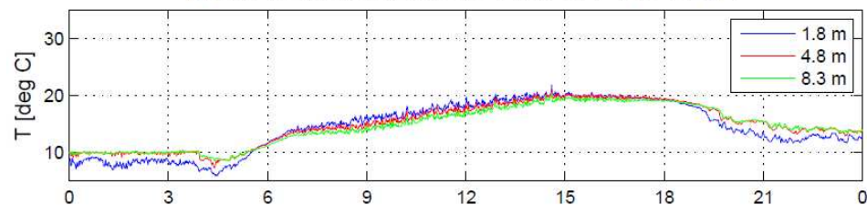
BLLAST Lannemezan site 1 flux GFI 19.06.2011
