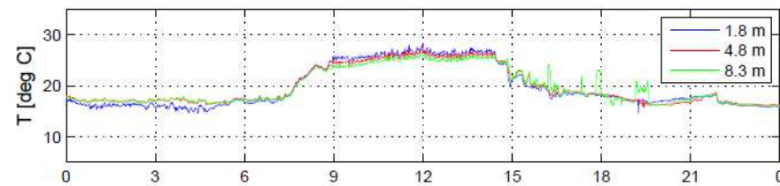
BLLAST Lannemezan site 1 flux GFI 03.07.2011
